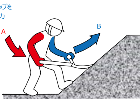
バラスコ1人作業 補助ハンドルを引き上げる力B+押す力A
